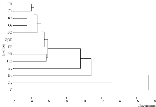
Рис. 3. Дендрограмма мер сходства населения мелких млекопитающих в разных биотопах г. Кишинева. Условные обозначения см. рис. 1
