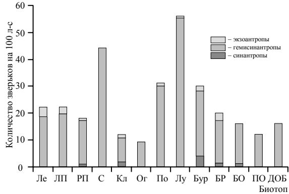
Рис. 1. Соотношение разных по склонности к синантропии групп мелких млекопитающих в биотопах г. Кишинева: Ле – леса, ЛП – ландшафтные парки, РП – регулярные парки, С – сады, Кл – кладбища, Ог – огороды, По – поля, Лу – луга, Бур – бурьяны, БР – берега рек, БО – берега озер, ПО – полосы отчуждения железных дорог, ДОБ – дворы овощных баз
