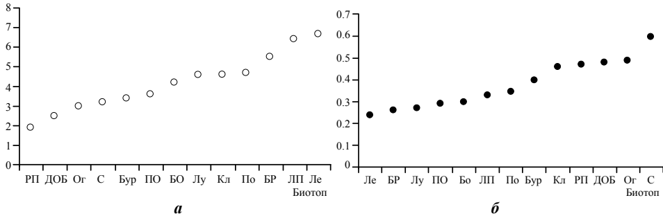
Рис. 2. Показатели индексов видового разнообразия (а) и концентрации доминирования (б) мелких млекопитающих на незастроенных территориях г. Кишинева. Условные обозначения см. рис. 1
